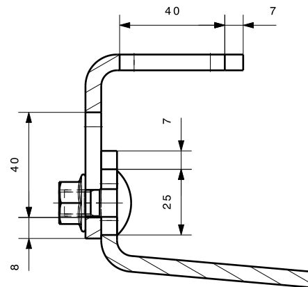
Schnitt A-A Maßstab: 1:2
